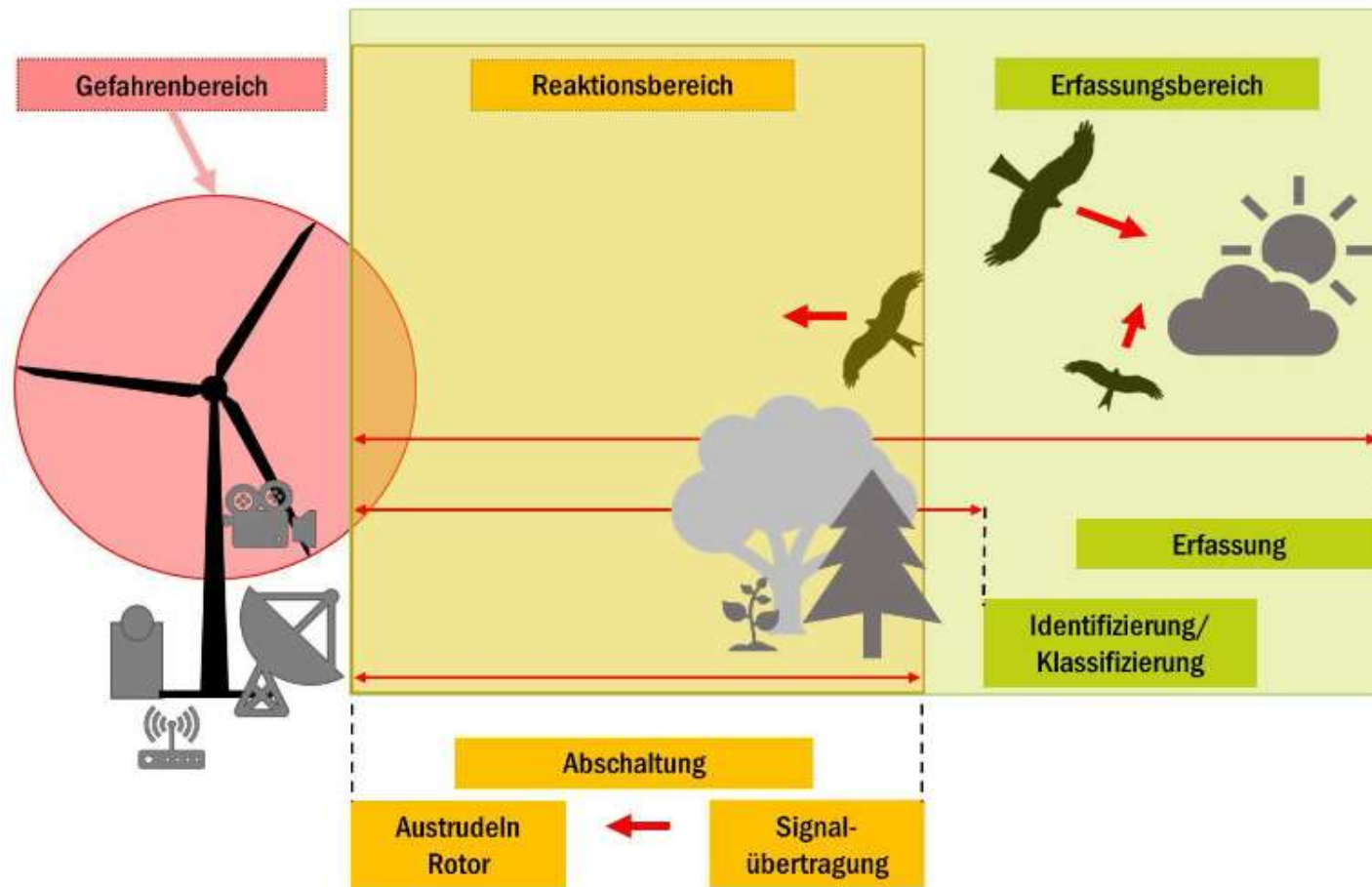
Abbildung 1: Schritte der technischen Detektion und Betriebsregulierung einer Windenergieanlage (schematisch; Quelle: KNE, verändert)
