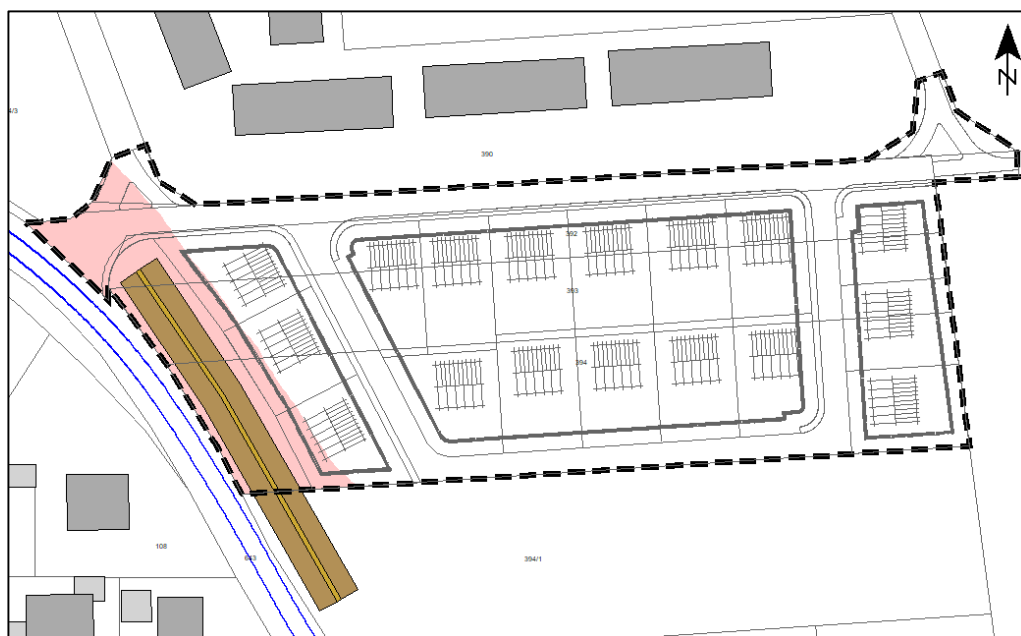
Abbildung 9 – Kennzeichnung Lüftungseinrichtungen mit Lärmschutzwall, Variante 2 (hellrot: Pegelwerte nachts > 50 dB(A)), Rechenhöhe 8 m ü. Gel.
