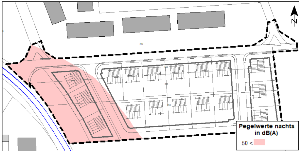
Abbildung – Kennzeichnung Lüftungseinrichtungen (hellrot: Pegelwerte nachts > 50 \text{ dB(A)} ), Rechenhöhe 8 m über Gelände
